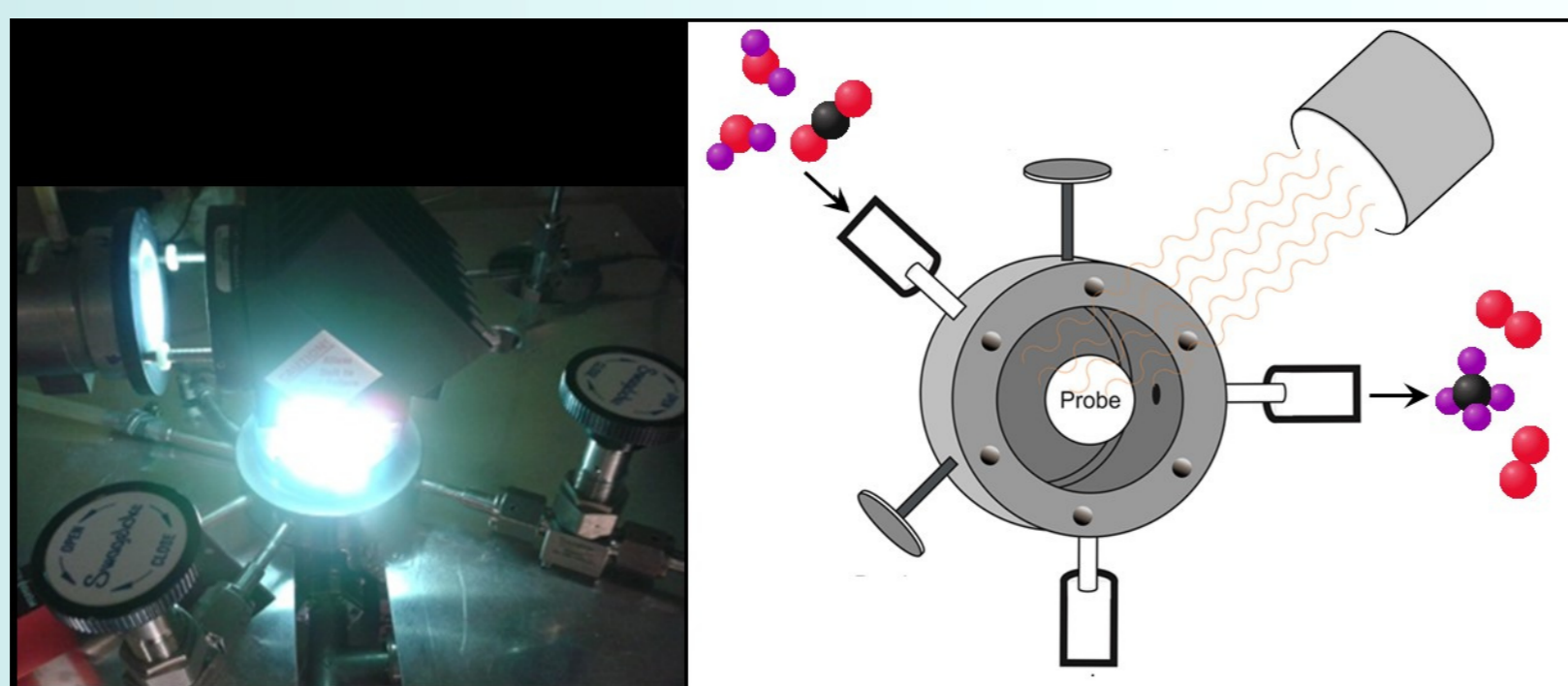
Photokatalytische CO 2 -Reduktion: Schematische Darstellung (rechts) und Bild des laufenden Gasphasenphotoreaktors (links).
