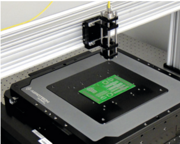
Fertigungseinrichtung zur Direktbelichtung von lichtempfindlichen Schichten mittels UV-Laserstrahl.
